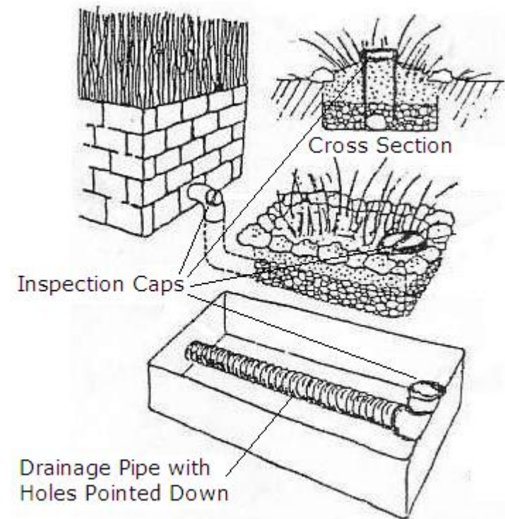
ET Treatment Beds
